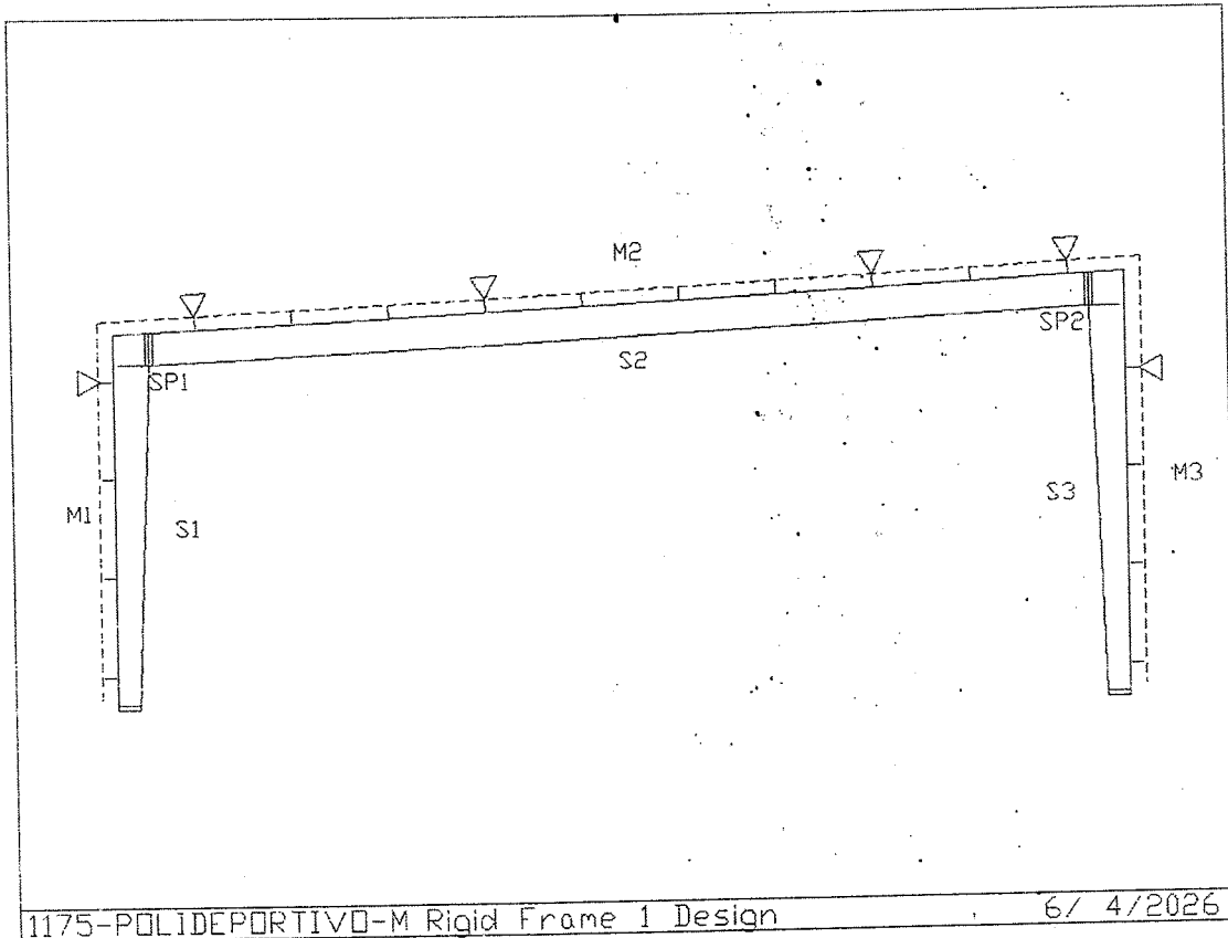
Pórtico típico
